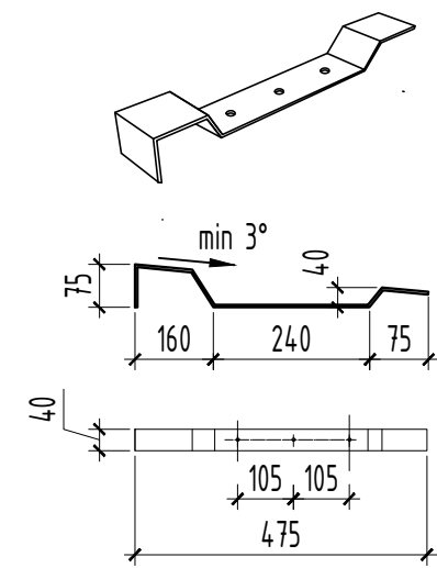
Козыль кровельный схема сгиба М 1:25
